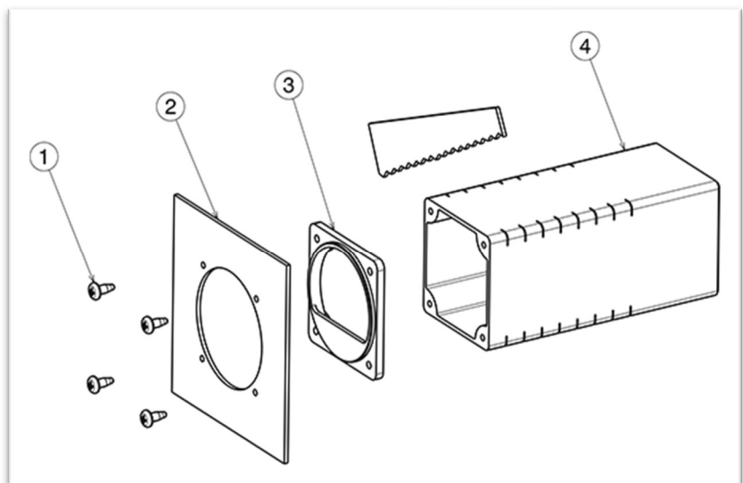
Abb.2: Technische Zeichnung Explosionszeichnung Anordnung I-Brett Ablage
